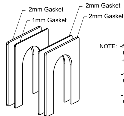
Gaskets
