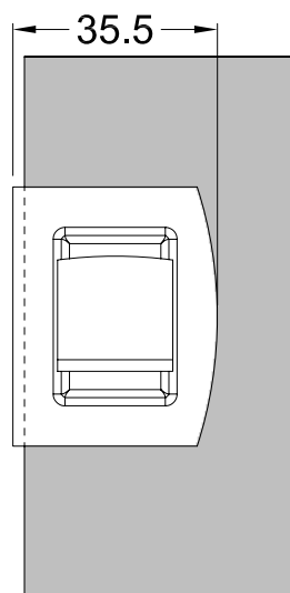
GK624(LH) Strike
