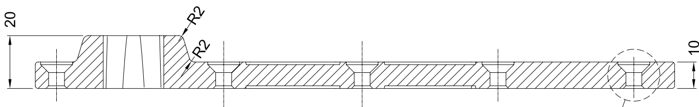
SECTION A-A
