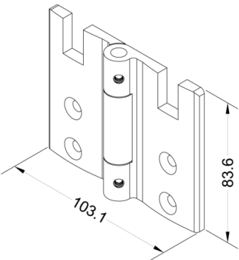
HN80 – Hinge (DRM80)
