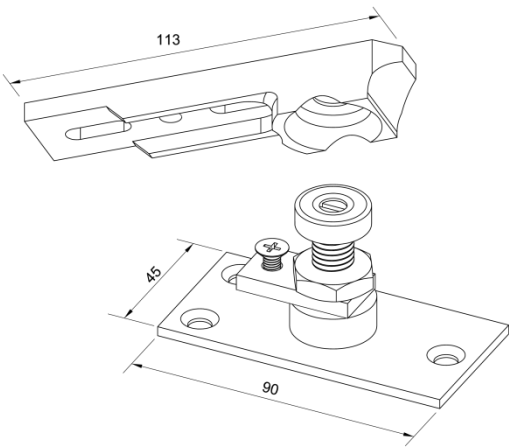
PD16- Bottom Pivot
