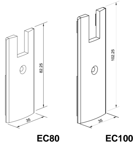
End Cap
