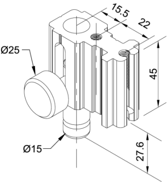
FB- Front Flush Bolt
