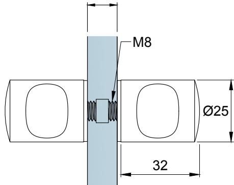
KH16 Ø25 Door Knob
