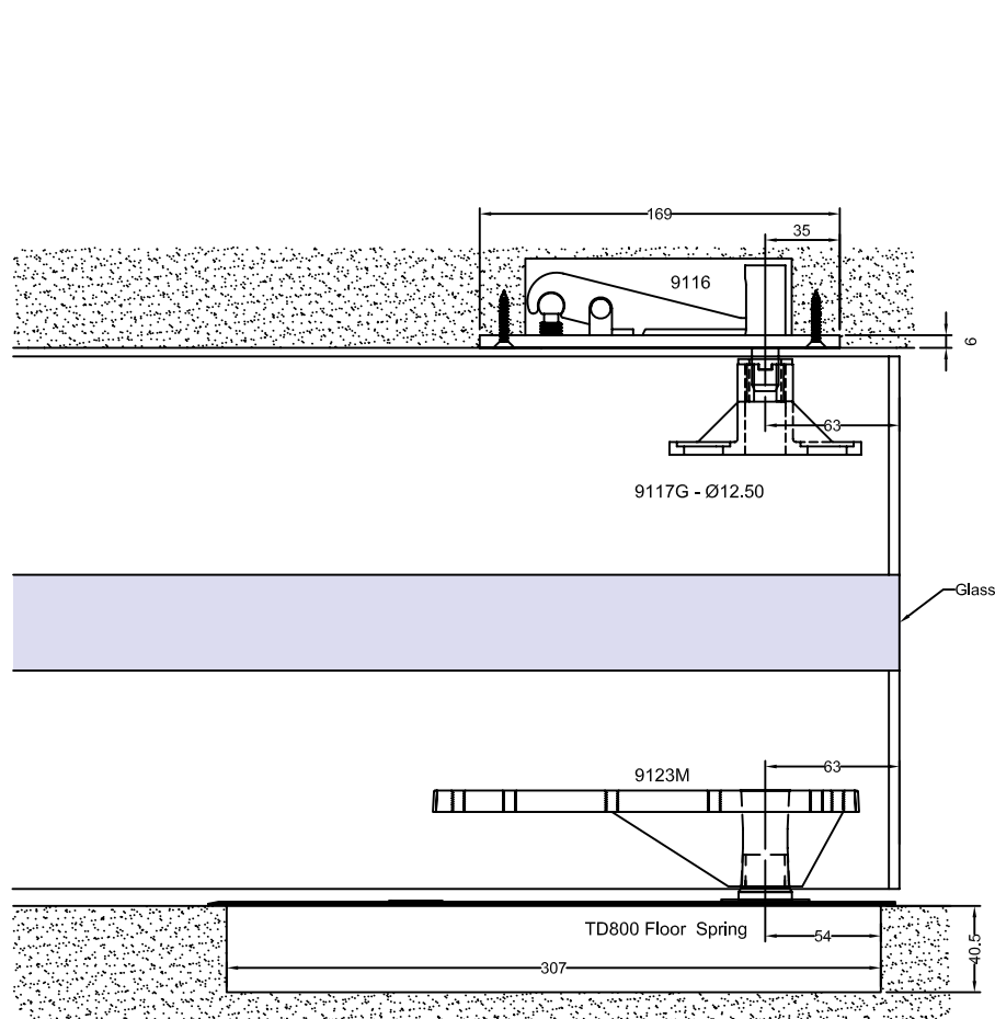
DRM100 Door Rails Elevation
