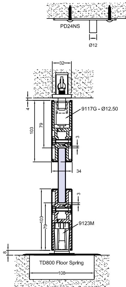
DRM100 Door Rails
