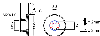
Point Stud (Adjustable)
