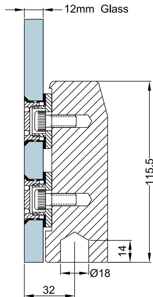
SECTION A-A
