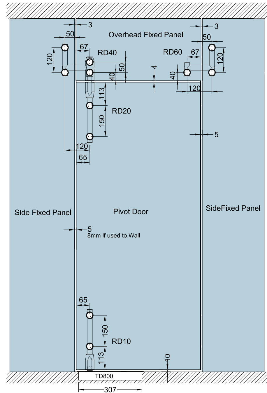
ELEVATION
