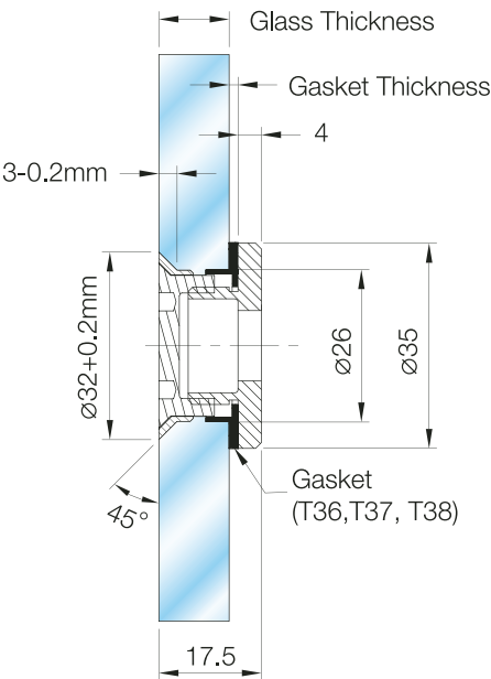
CSA-Countersunk Point Stud (Adjustable)
